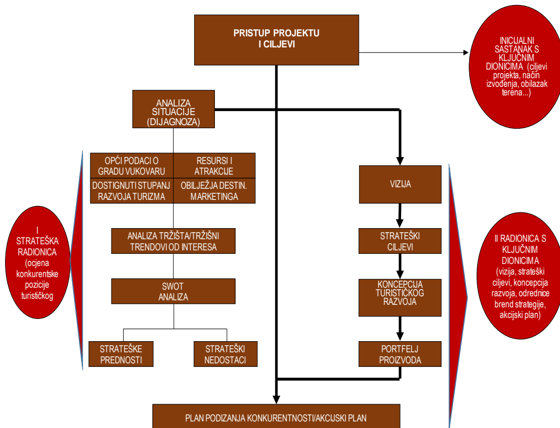
Slika 1.5.1. Struktura dokumenta
