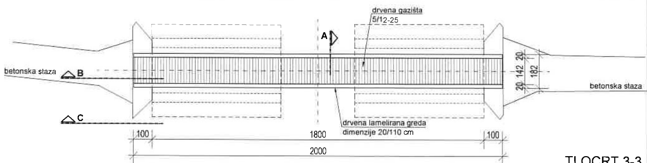
TLOCRT 3-3
