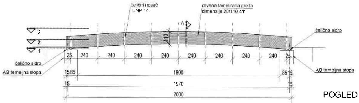
PRESJEK B-B
